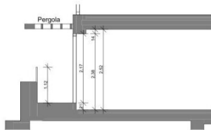
Schnitt 2/67 A
