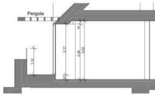
Schnitt 1/71 A
