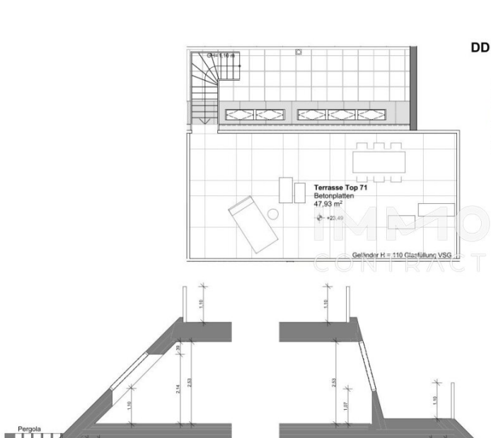
Schnitt 2/71 A
