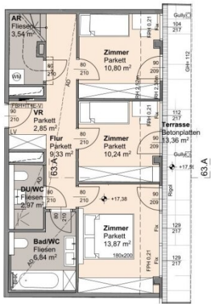
Grundriss 1.Dachgeschoss
