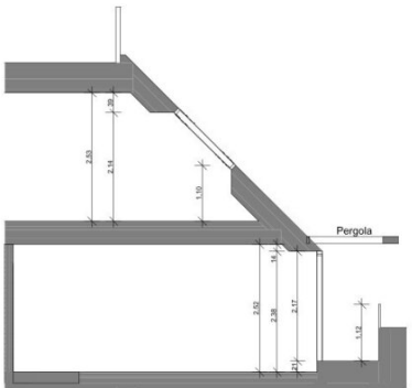
Schnitt 2/63 A
