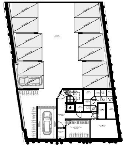
UNTERGESCHOSS M = 1:200
