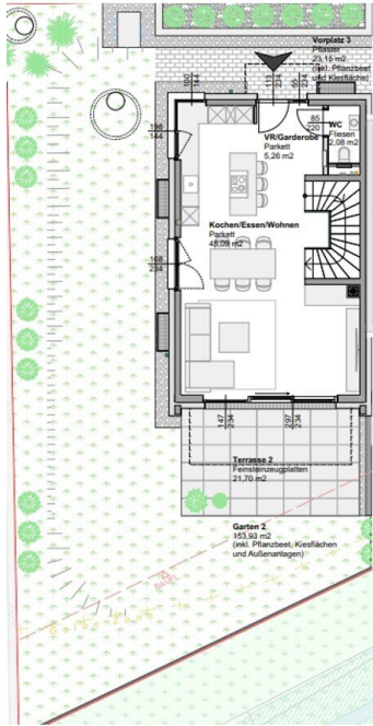
Erdgeschoss
