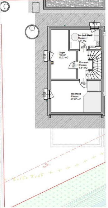
Kellergeschoss
