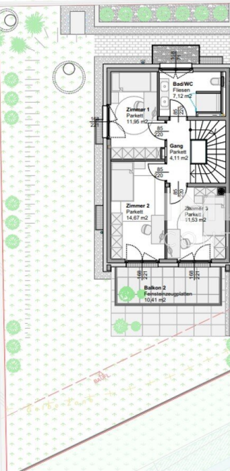
1. Obergeschoss
