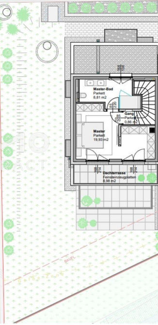
Dachgeschoss
