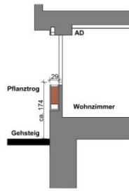
Fassadenschnitt
