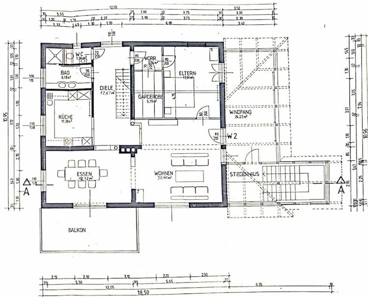
OBERGESCHOSS
