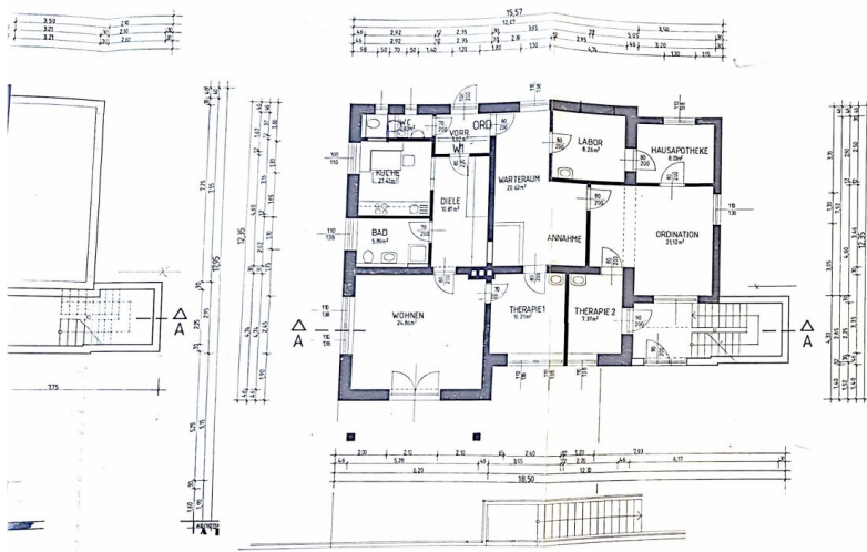
ERDGESCHOSS
