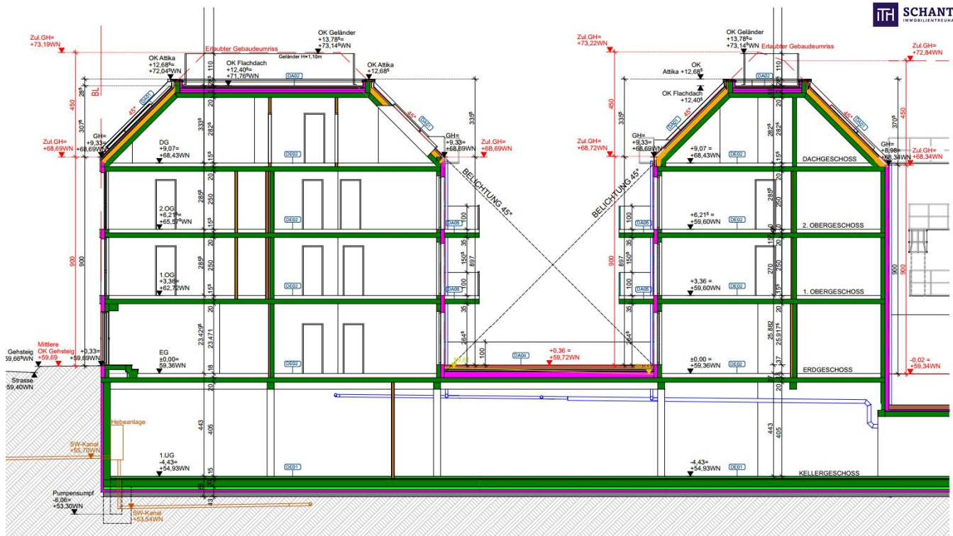
SNITT A-A 1:100
