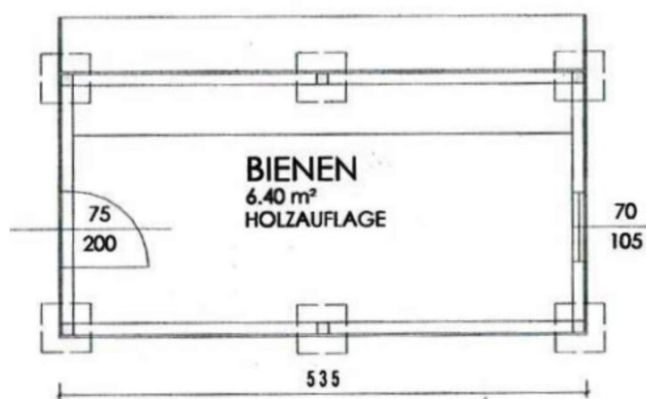
GRUNDRISS BIENENHÜTTE
