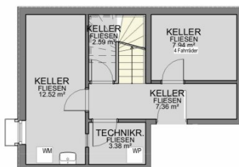
KELLER
