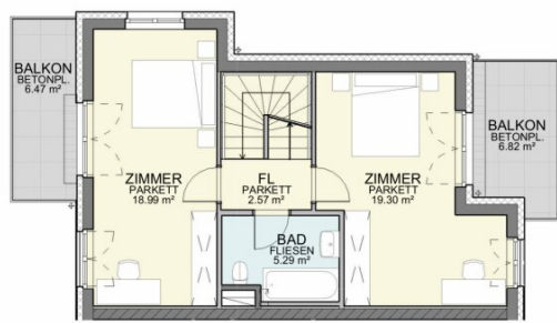
1.OBERGESCHOSS
