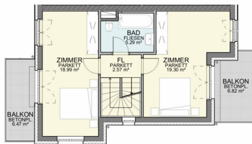
1.OBERGESCHOSS
