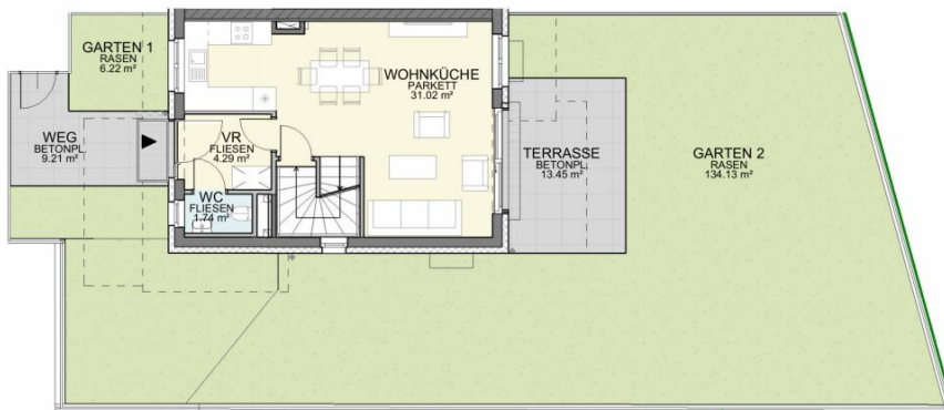
ERDGESCHOSS
