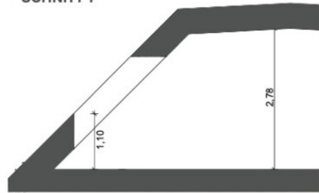
SNITT 1
