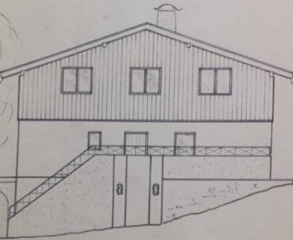
NORD-OST ANSICHT
