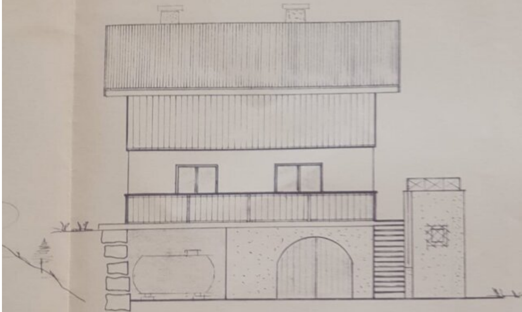
SÜD-OST ANSICHT
