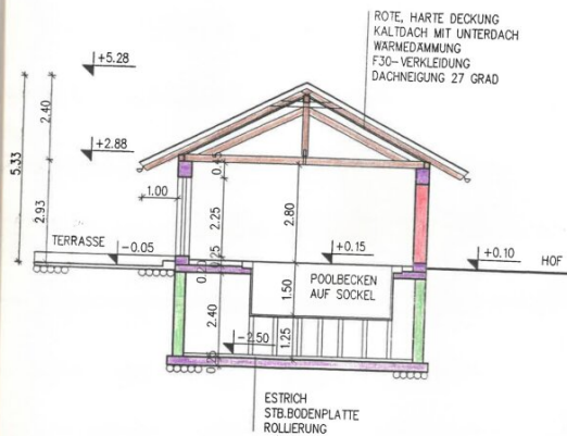
SCHNITT 3 - 3
