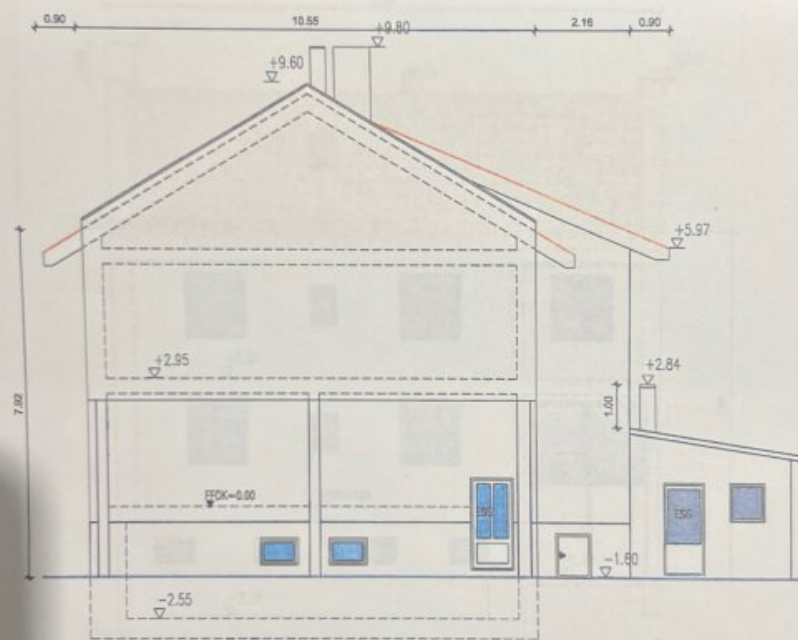
ANSICHT - OST M. 1:100
