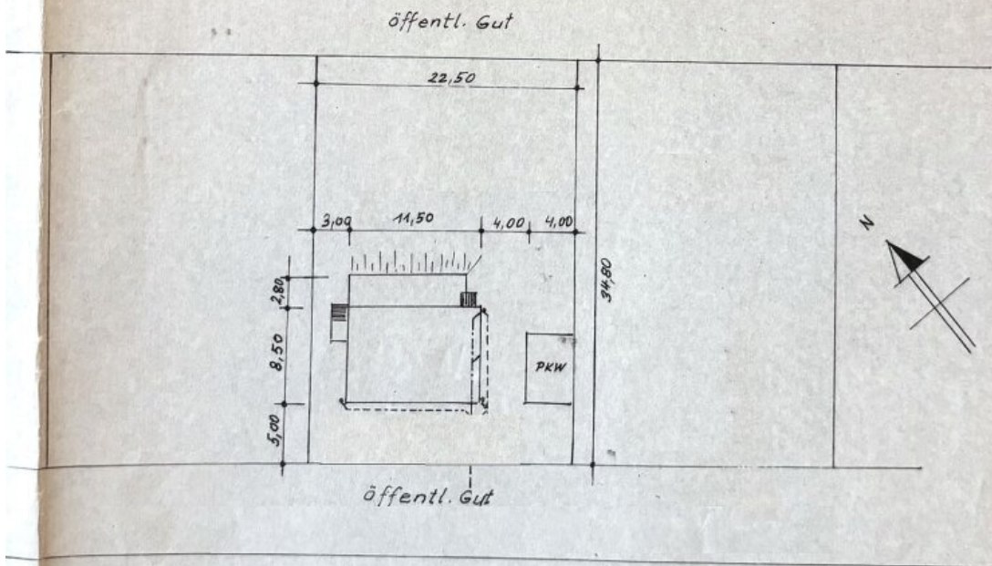
LAGEPLAN M 1:500
