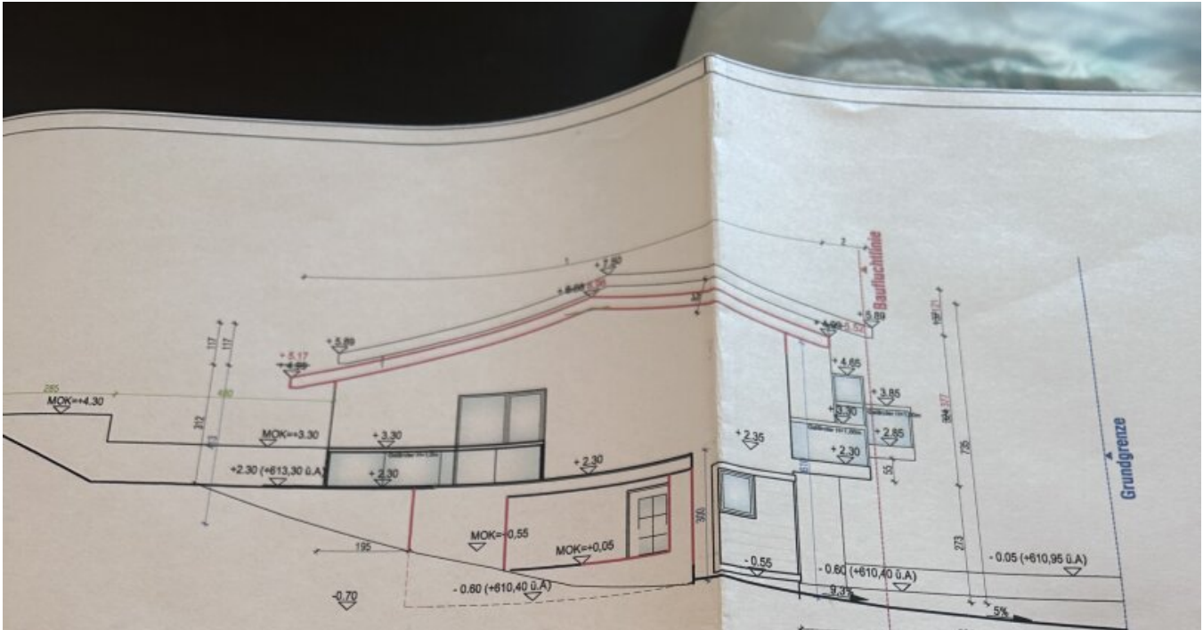
ANSICHT NORD
