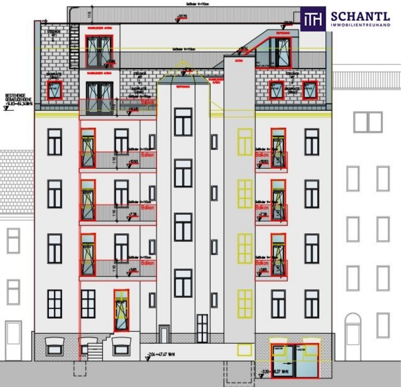
ANSICHT HOF
