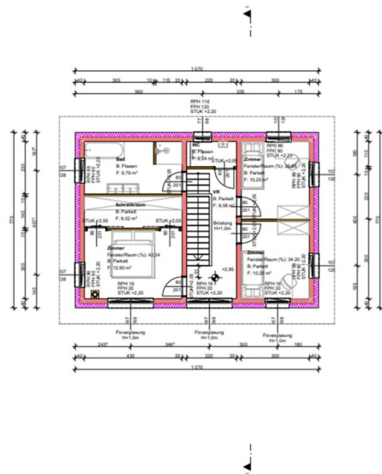
1. Obergeschoss 1:100
