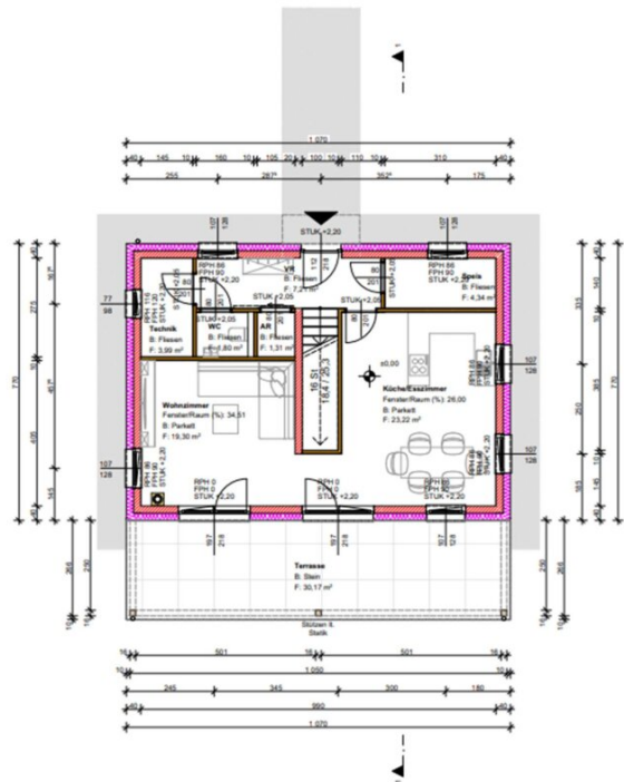
0. Erdgeschoss 1:100
