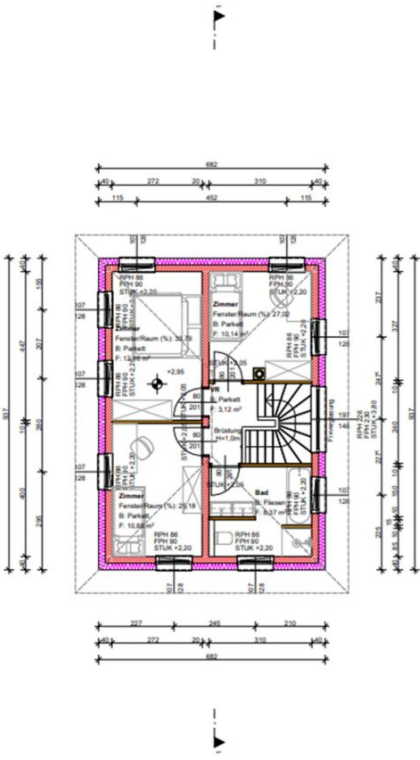
1. Obergeschoss 1:100
