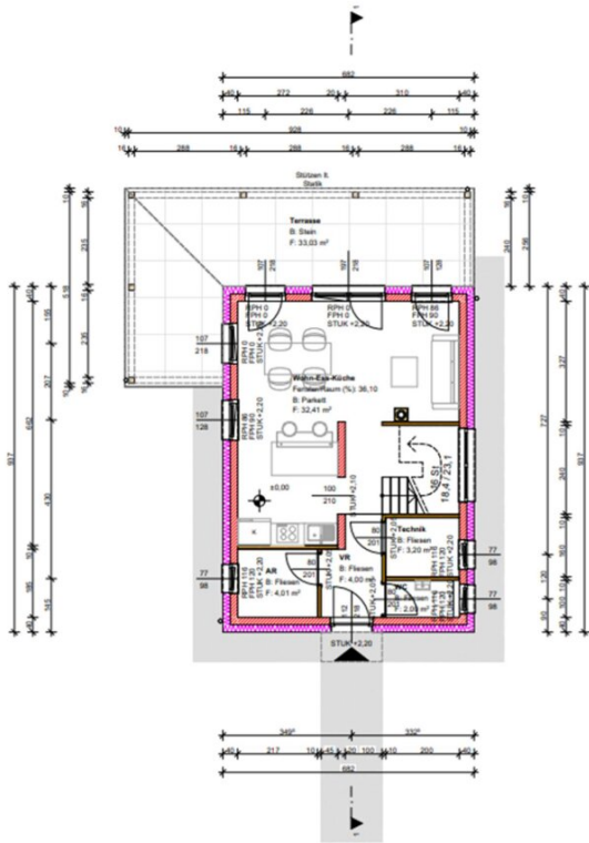
0. Edgesschoss 1:100
