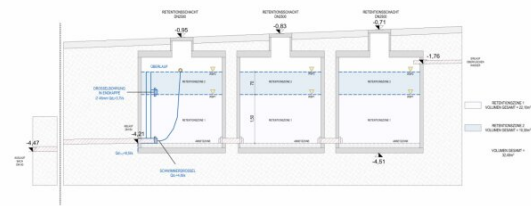
RETENTIONSSTUFE 01 M 1:500
