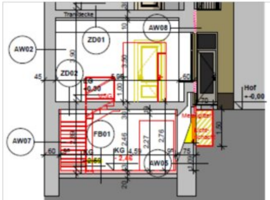
SCHNITT S01:
