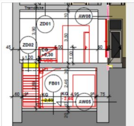
SCHNITT S05:
