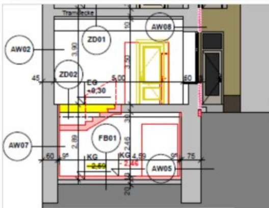
SCHNITT S02:
