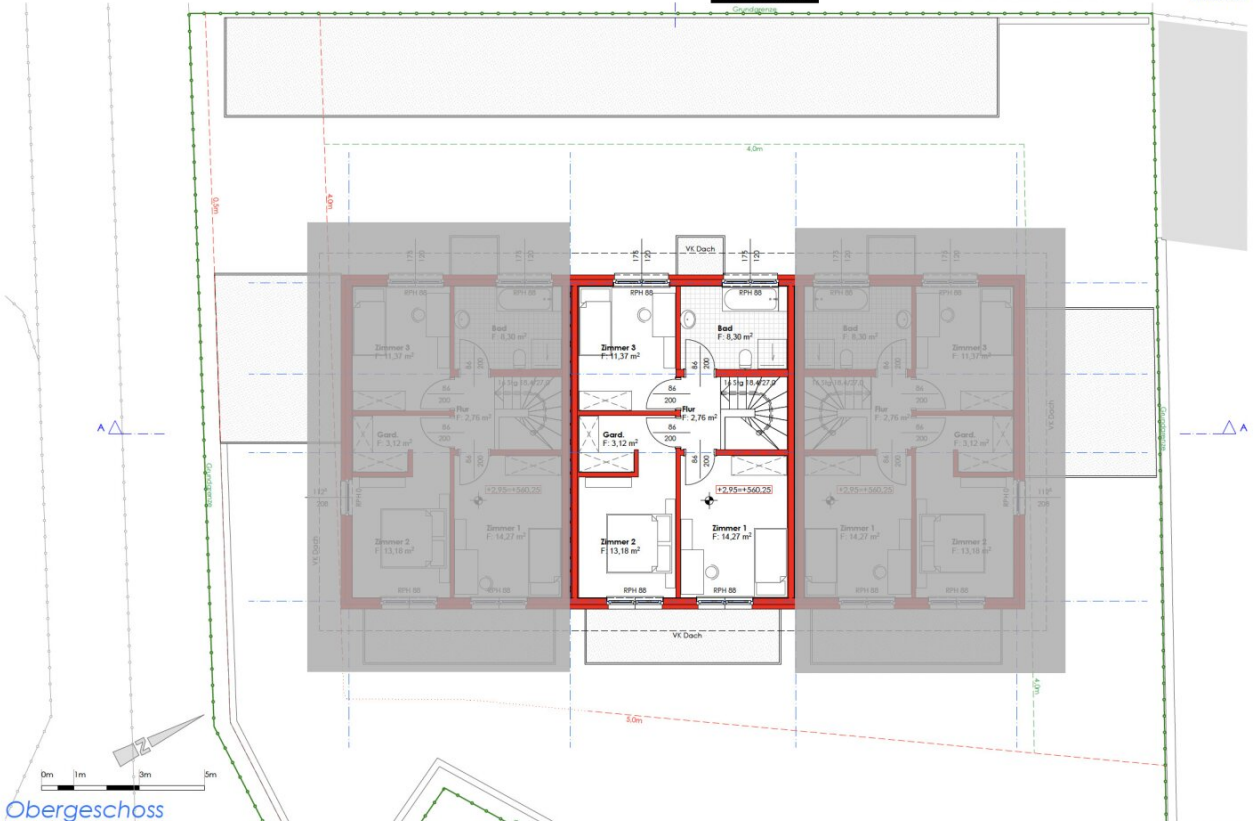
GRUNDRISS 1:100
