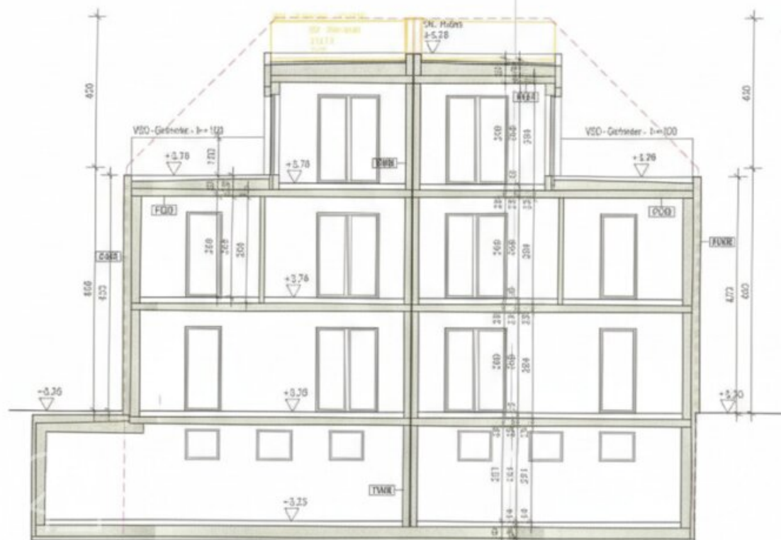
Schnitt C-C
