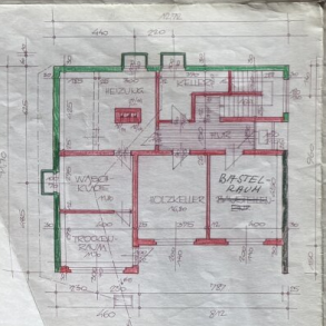
TIERPARTEREGRUNDRISS
