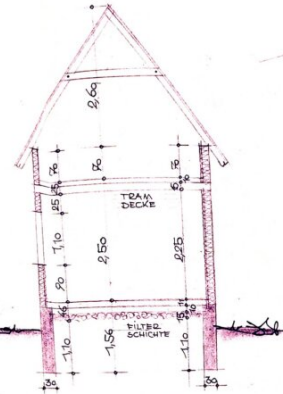
SCHNITT AB
