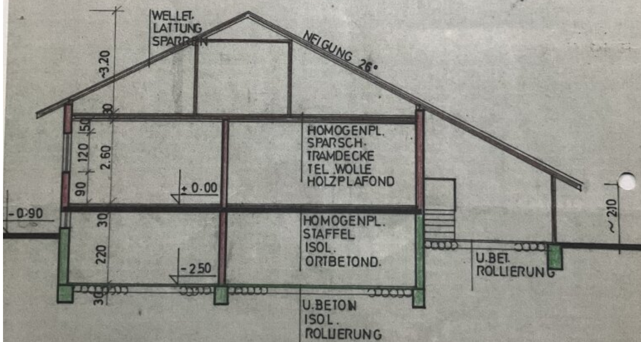
SCHNITT A-A
