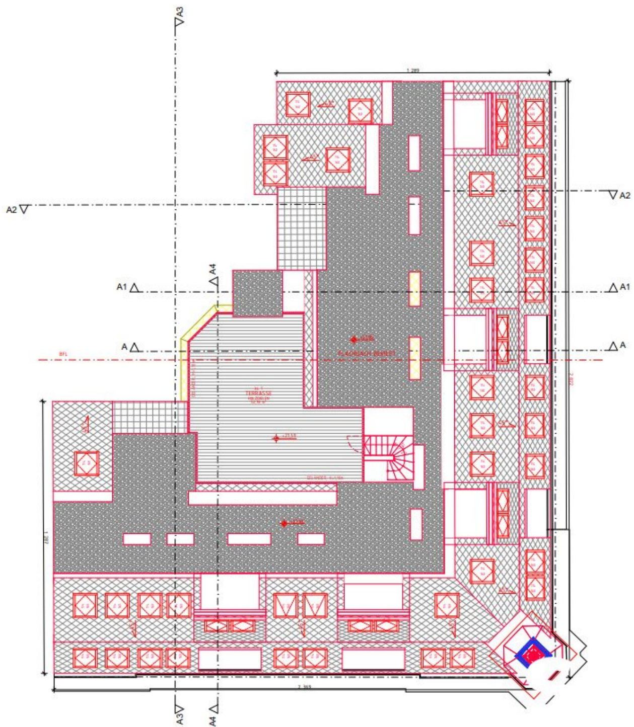
DACHDRAUFSICHT
