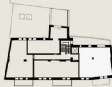
SASSMANNHAUS 2.OG
