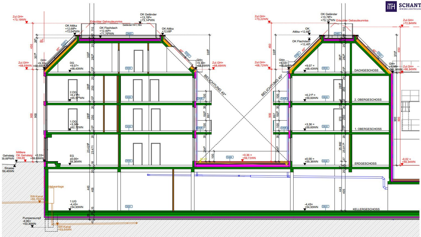
SNITT A-A 1:100
