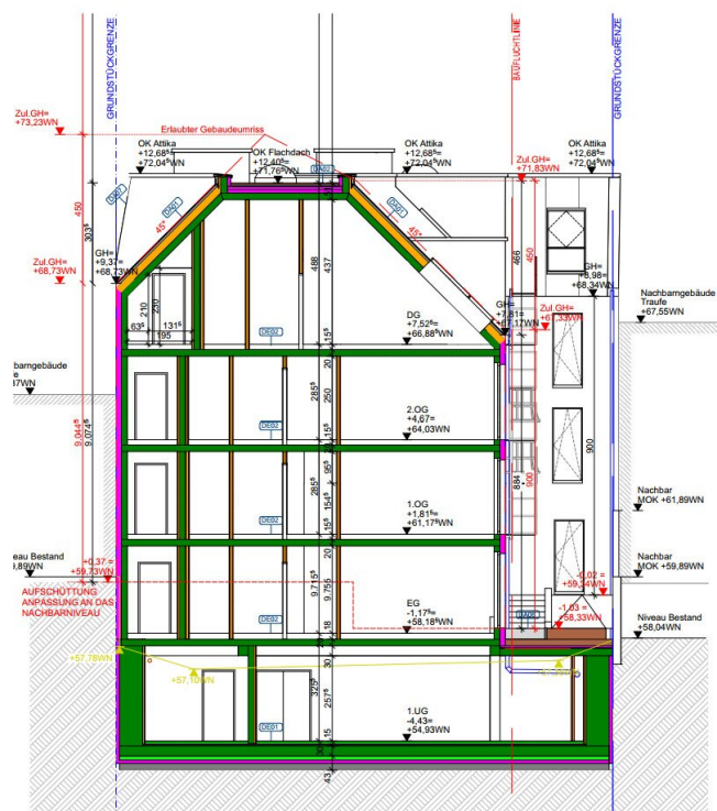
SCHNITT B-B 1:100
