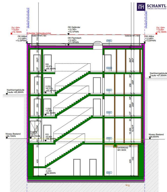
SCHNITT D-D 1:100
