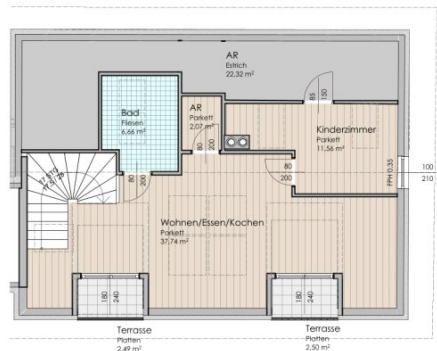
Grundriss DG
