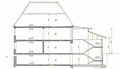
SCHNITT A-A
