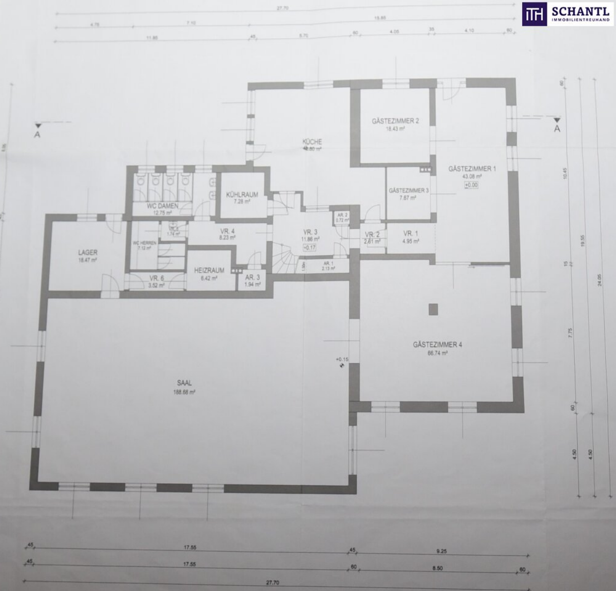
GRUNDRISS EG
