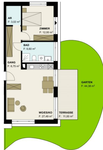
Grundriss Wohnung
