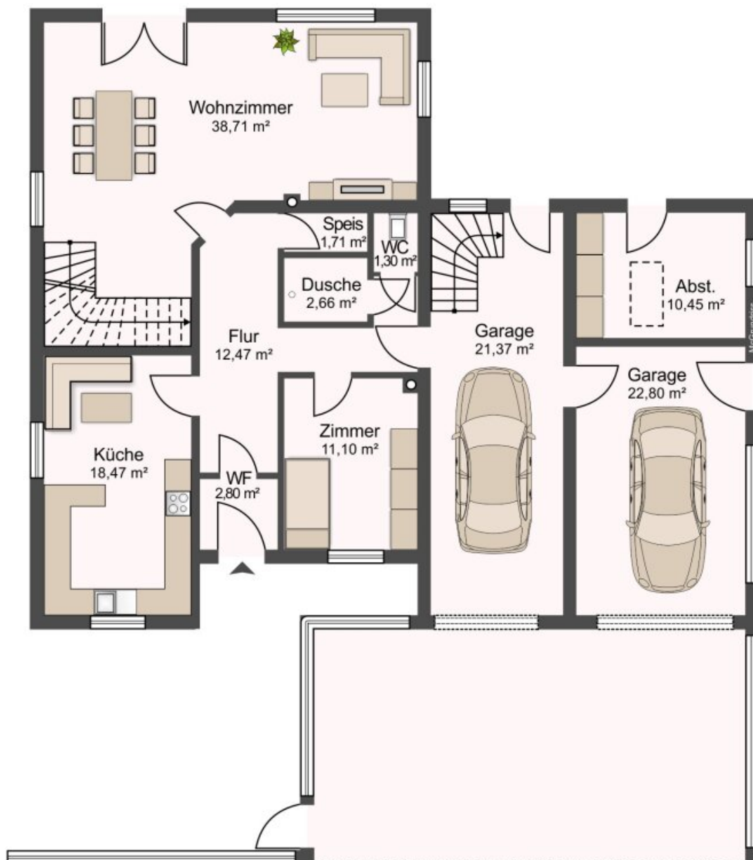
Erdgeschoss
