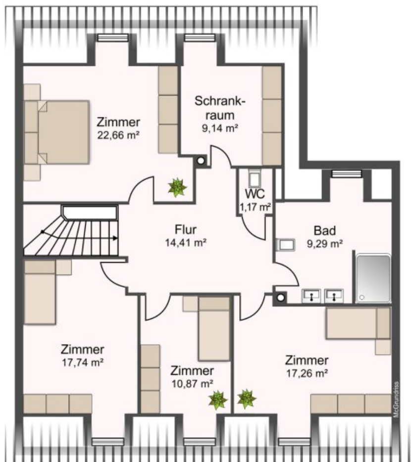
Obergeschoss
