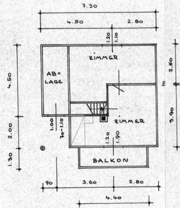
OBERGESCHLOSS
