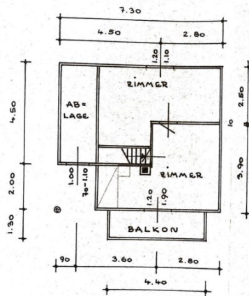
OBERGESCHOSS
