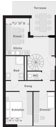
Dachgeschoss
