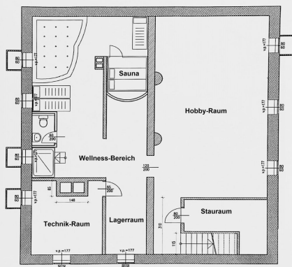
Grundriss Villa Untergeschoss
