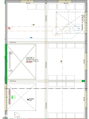
Top 4.1 - Erdgeschoss
