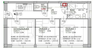
Top 5 - Obergeschoss
