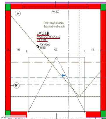
Top 2 - Erdgeschoss
