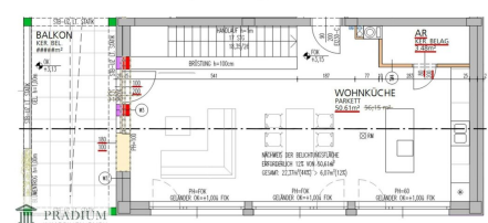
Top 5 - Obergeschoss
