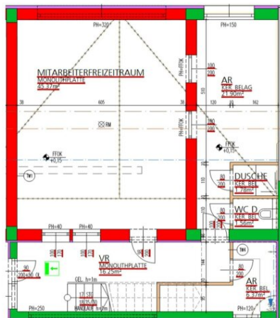
Top 3 - Obergeschoss
