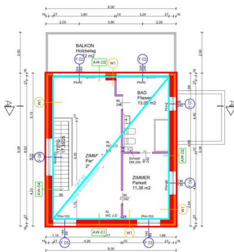
00-EA GRUNDRISS OG 1:100
