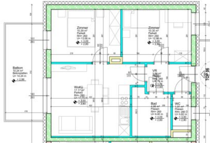
Planausschnitt 2.OBERGESCHOSS - Wohnung Planstand = Ausführungsplan M: 1:100
