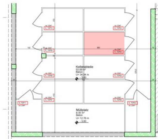
Planausschnitt KELLERGESCHOSS - Abteil TOP 06 - OST Planstand = Ausführungsplan M: 1:100
