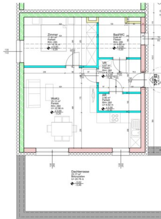
Planausschnitt 1.OBERGESCHOSS - Wohnung Planstand = Ausführungsplan M: 1:100
