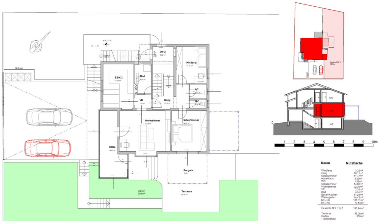
Top 1 Erdgeschoß
