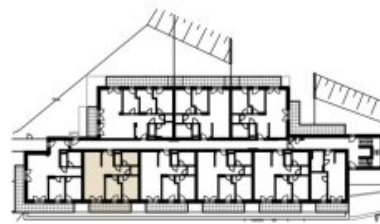
GRUNDRISS BK 03
