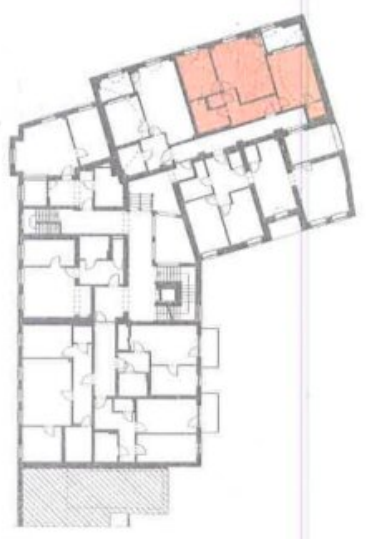
ÜBERSICHT - OG
