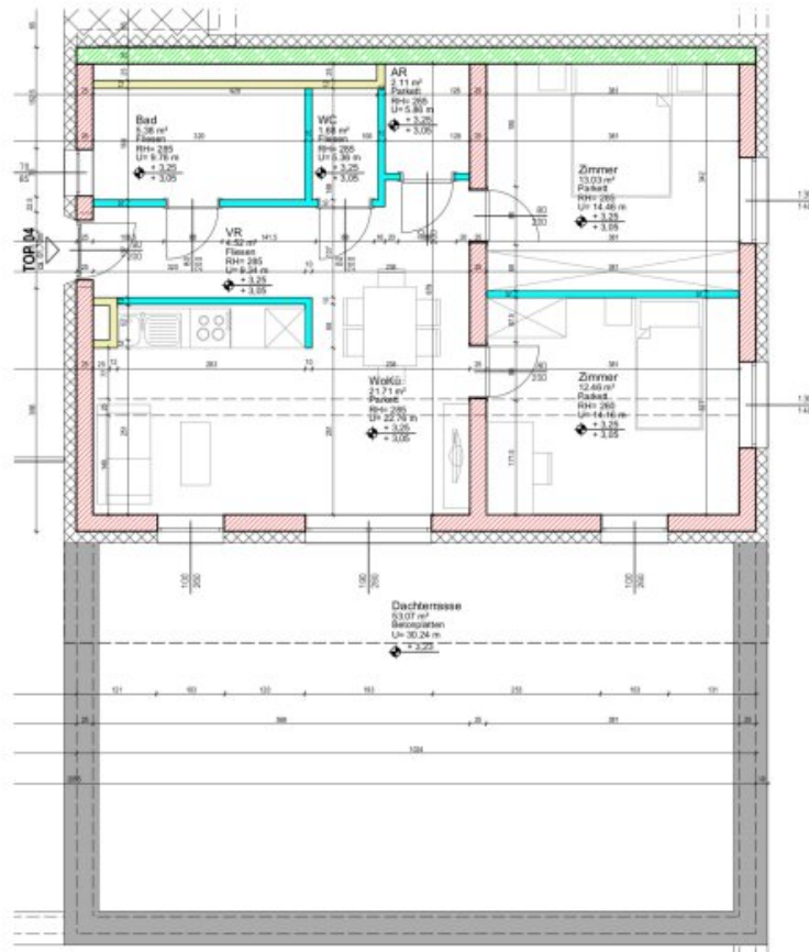
Planausschnitt 2.OBERGESCHOSS - Wohnung Planstand = Ausführungsplan M: 1:100
