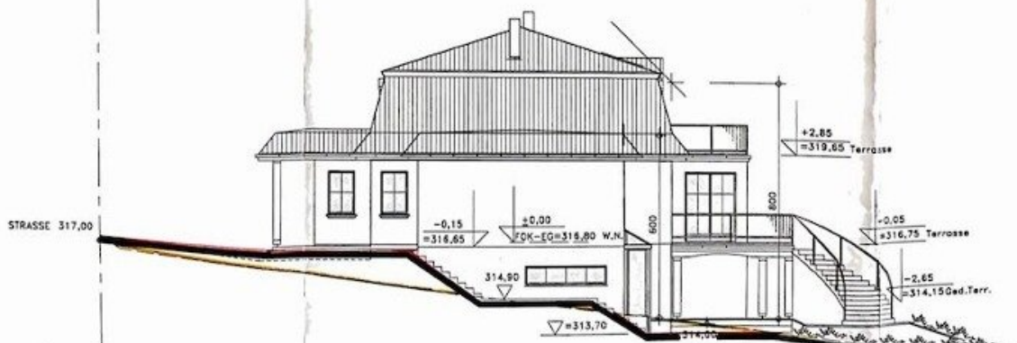
WEST-ANSICHT
