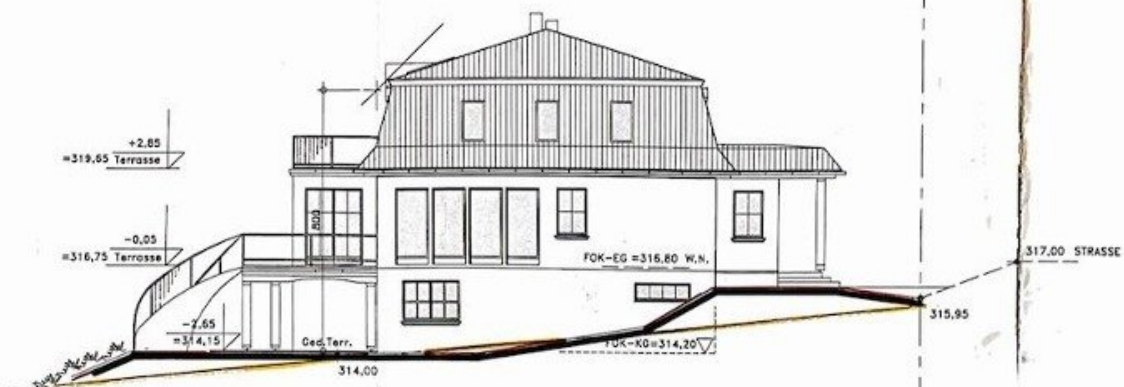
OST-ANSICHT
