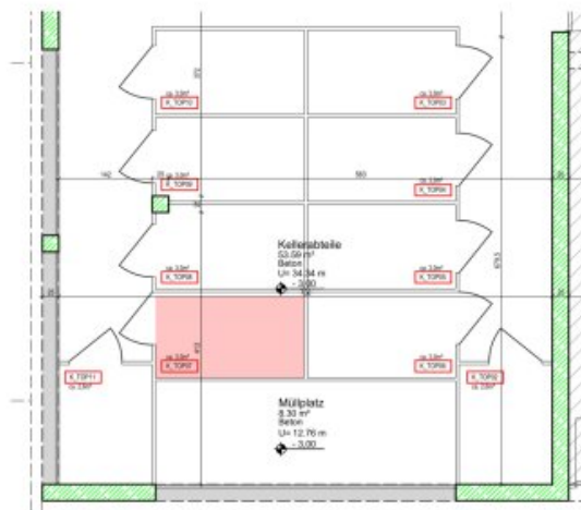
Planausschnitt KELLERGESCHOSS - Abteil TOP 07 - OST Planstand = Ausführungsplan M: 1:100
