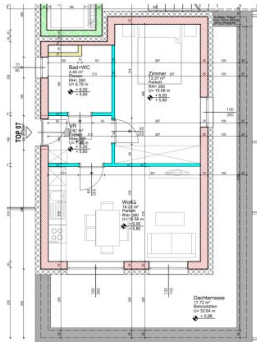
Planausschnitt 3.OBERGESCHOSS - Wohnung mit Dachterrasse Planstand = Ausführungsplan M: 1:100
